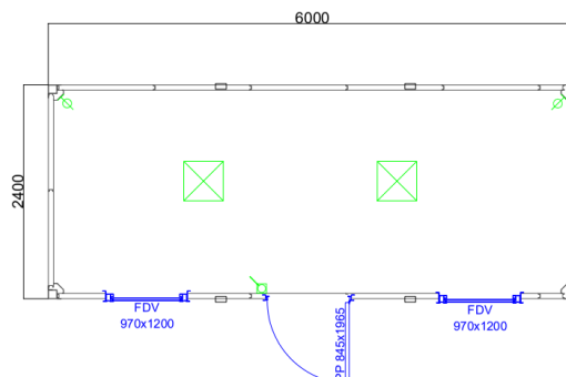
Figure 2 : Aperçu des dimensions
