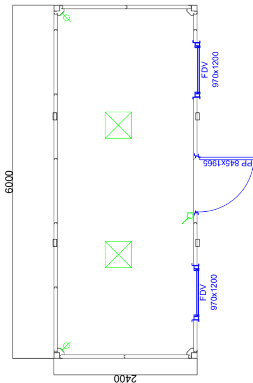
Figure 3 : Dimensions du module O60
