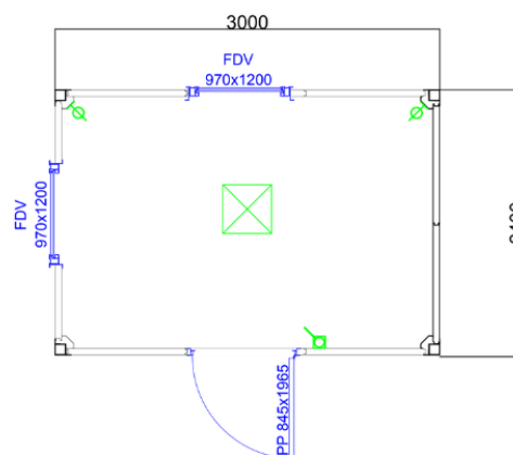
Figure 2 : Aperçu des dimensions
