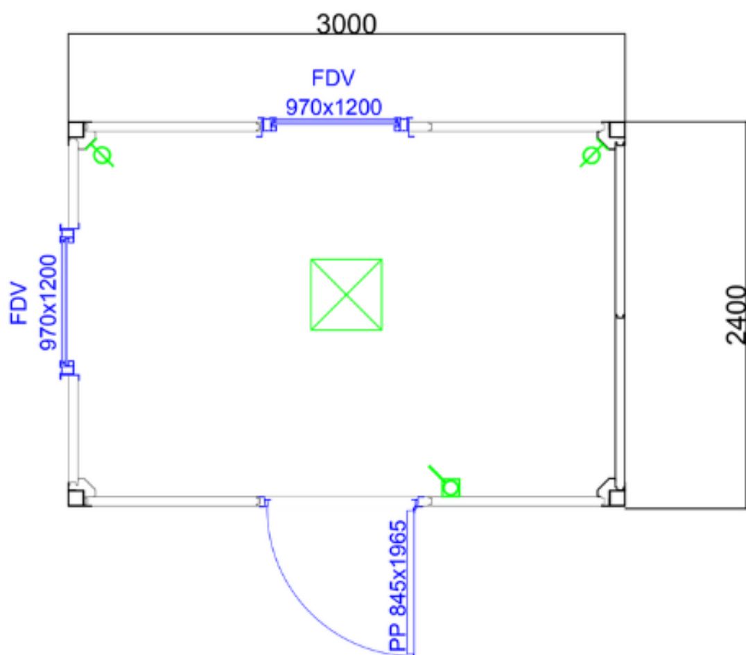
Figure 3 : Dimensions du module O30
